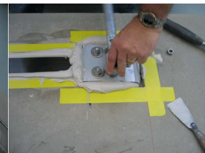
Die 4 Halteschrauben werden von Hand angezogen
