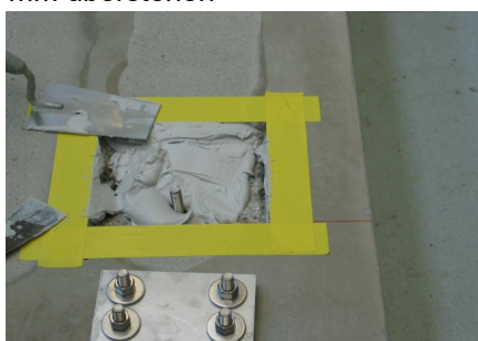
Die Aussparung wird mit dem Epoxidkleber verfüllt; das Gewinde muss ggf. anschließend gereinigt werden
