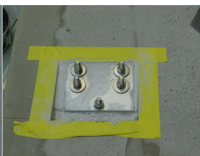
Ist eine Vielzahl an Endverankerungen zu montieren, kann die Grundplatte in die Aussparung gepresst und die Schrauben leicht angezogen werden
