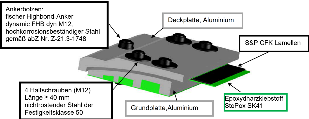
Bild 1: Aluminiumendverankerung Schematische Darstellung
