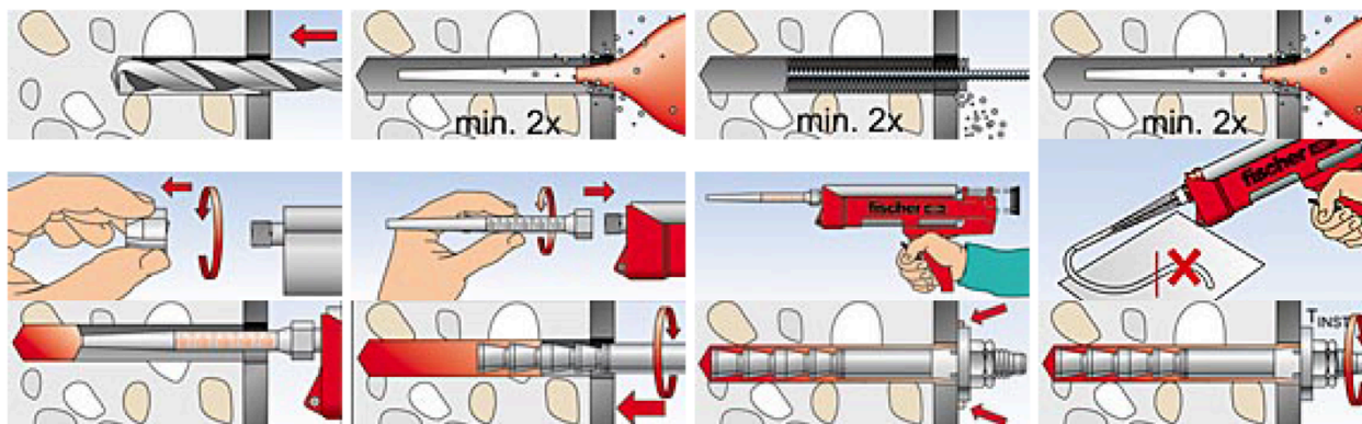
Bild 16: Setzen des Highbond-Ankers dynamic FHB dyn nach Z-21.3-1748
